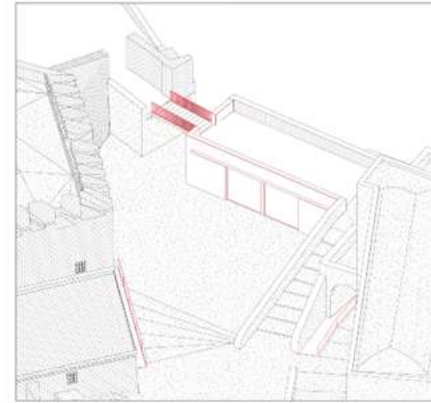
SCHEMI ASSONOMETRICI
